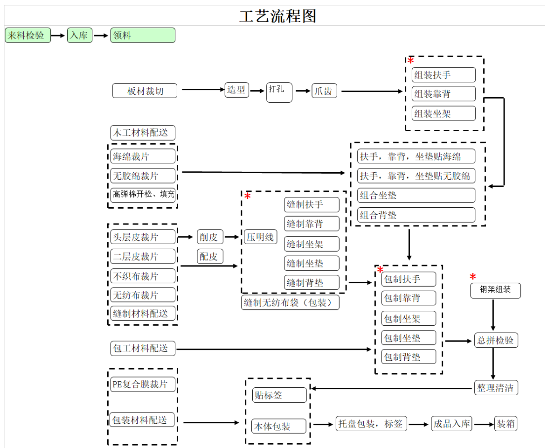
图 3.3 沙发工艺流程图
